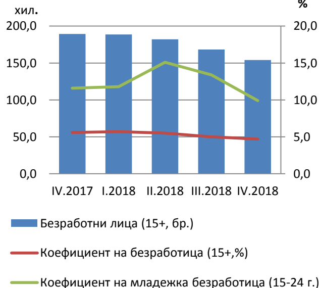
Фиг. 2 Безработица
