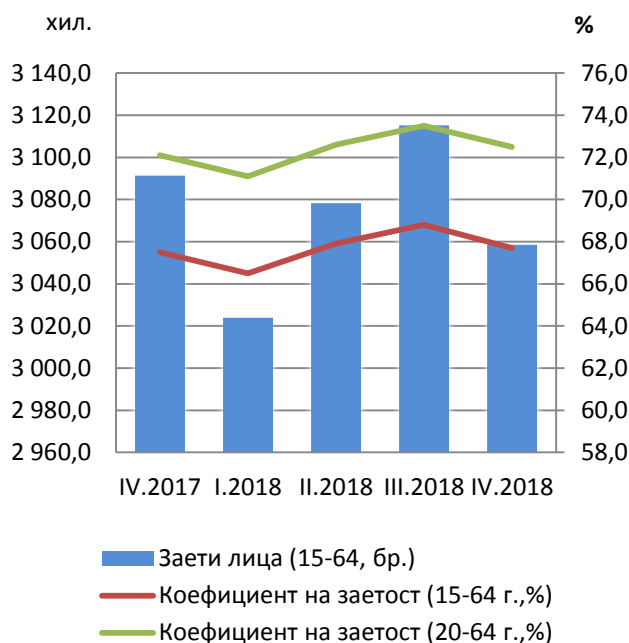
Фиг. 1 Заетост
